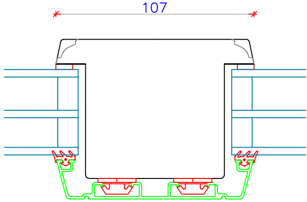
Lodret Spændestykke
