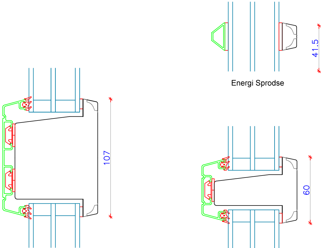
Vandret Spændestykke
