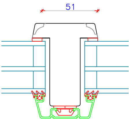
Lodret Sprodse
