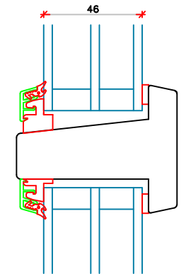
Vandret sprosse
